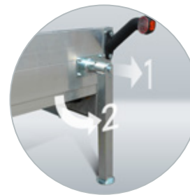
Enhåndsbetjente støttebein
