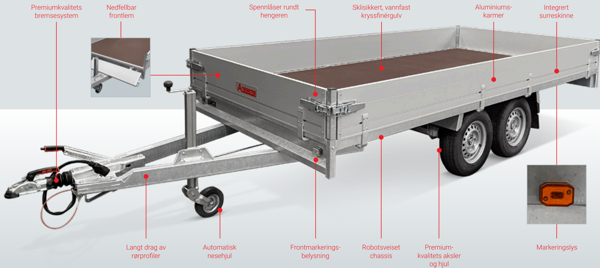
Lemmer kan slås ned under gulvet. Skadefri lasting og lossing
